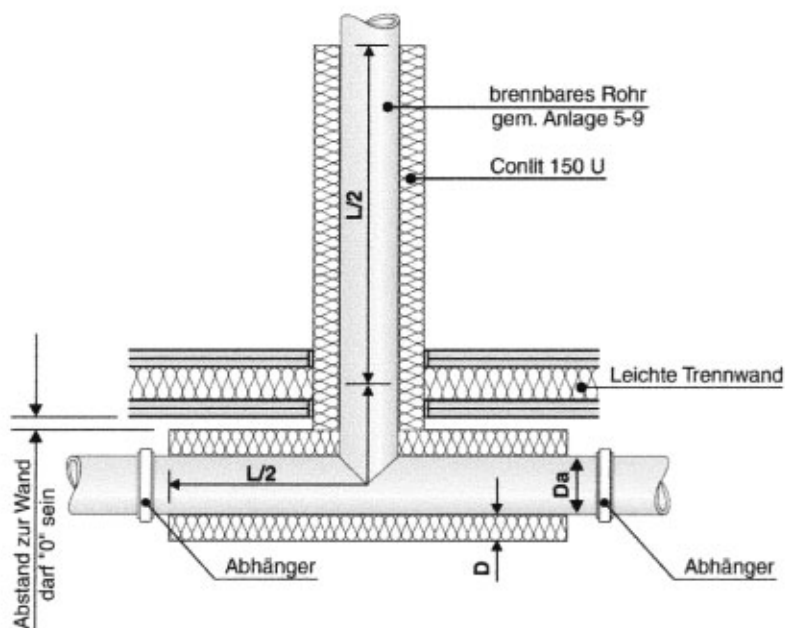
Prinzipskizze für Wand bei T-Stücken
