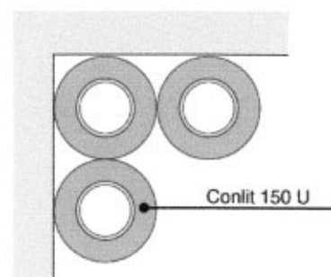
Prinzipskizze für Abstandsregelung bei Wand
