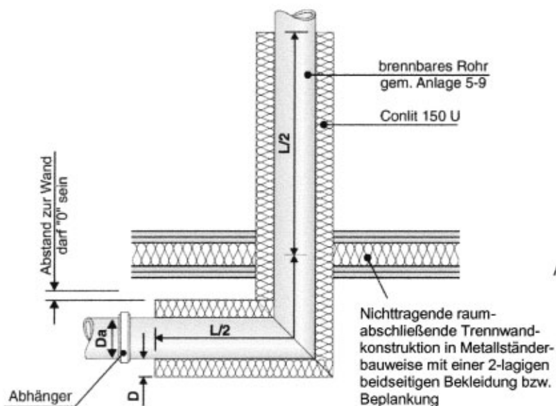
Prinzipskizze für Wand bei 90°-Bögen
