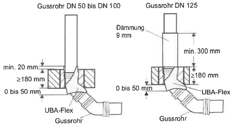
Rohrwerkstoff Gussrohr
