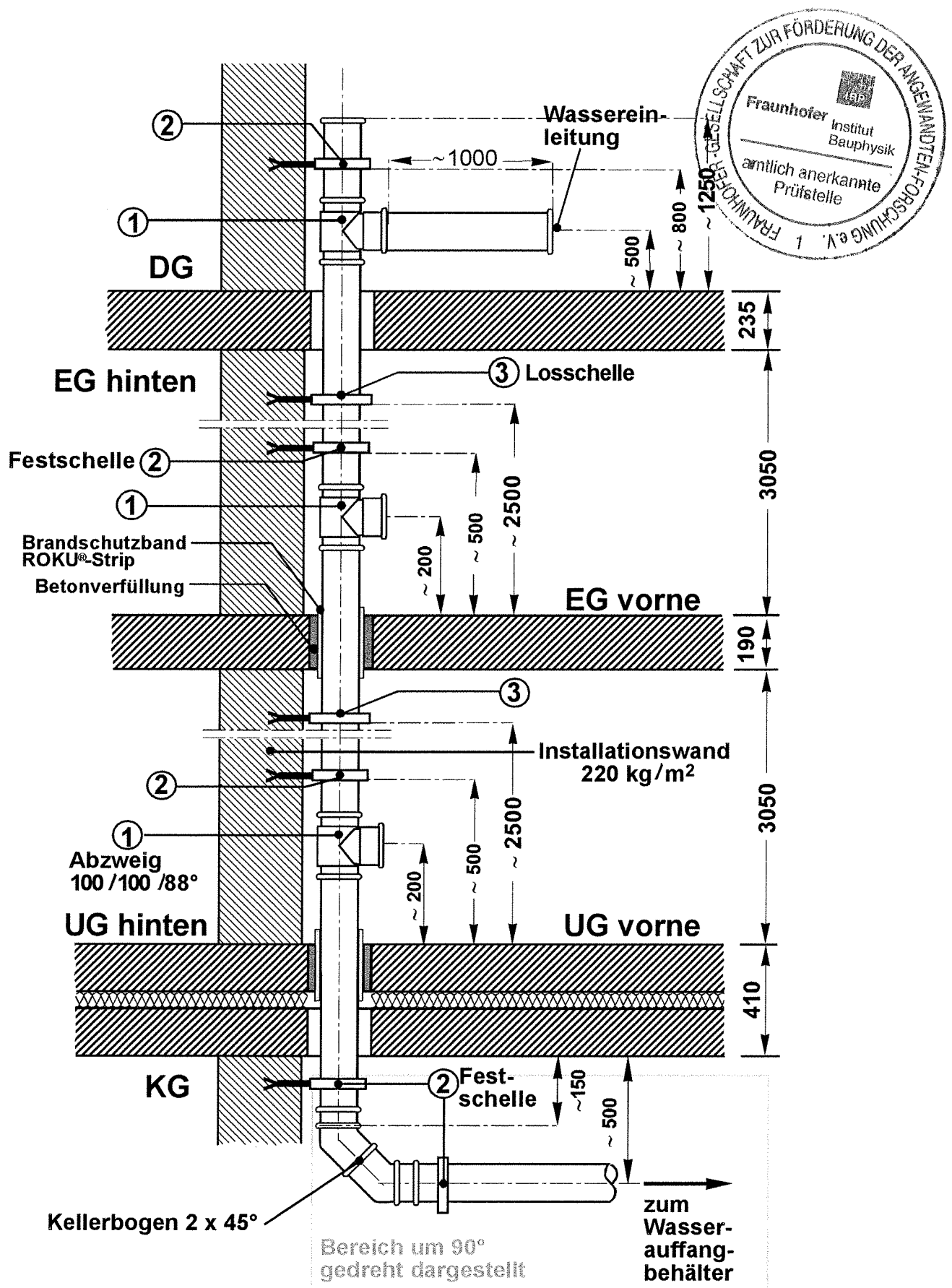
Bild 3 Fa. Rolf Kuhn. Installationsplan für alle Versuchsaufbauten. Die Rohrschellen waren bei allen Messungen an derselben Stelle angebracht. Bei den Messungen wurde das Brandschutzband "ROKU®-Strip" bzw. "ROKU®-Strip L 110" bzw. "ROKU®-Strip L 110 mit doppelseitigem Schaumstoffklebeband" in den Deckendurchbrüche EG/UG und UG/KG angebracht. Alle Maße in mm, Darstellung nicht maßstabsgerecht.
