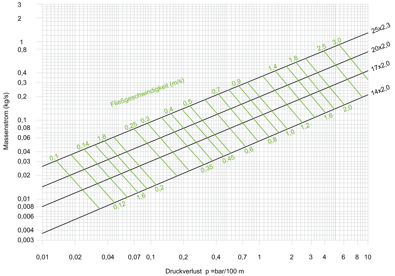
Druckverlust-Diagramm Heizrohr PE-Xa
