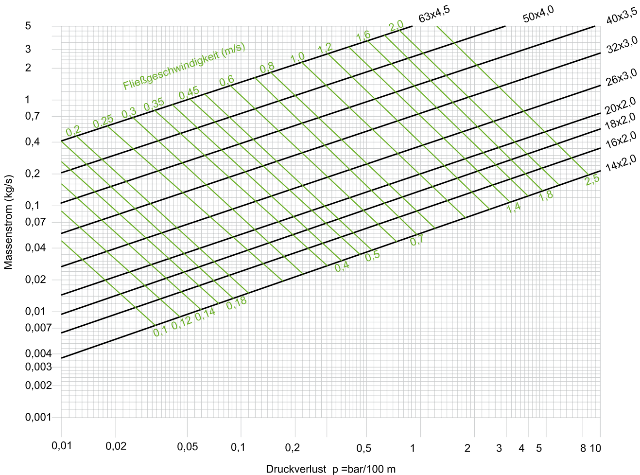
Druckverlust-Diagramm ZEWO Metallverbundrohre Heizung
