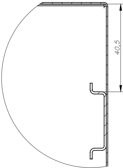
Detailausschnitt BQ Maßstab 1:1
