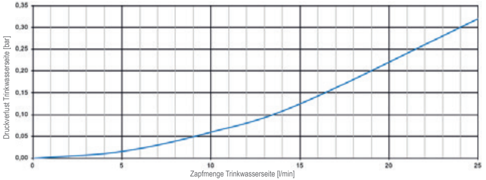
Druckverlust Trinkwasserseite eco 25 (sekundär)
